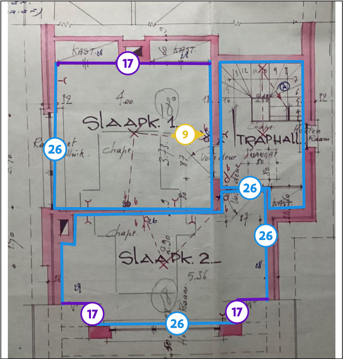
Legende van plan 1.3: Grondplan verdieping
